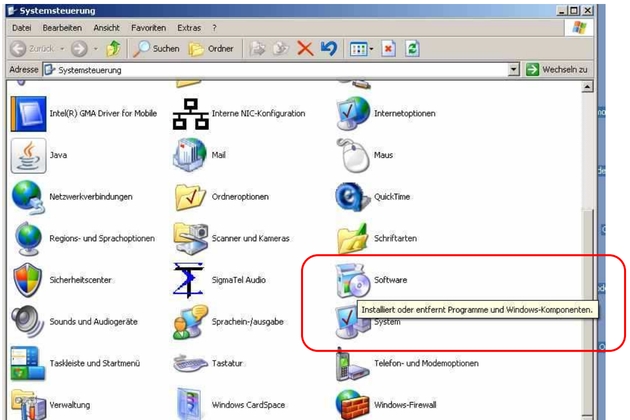
Abbildung 2 Ordner Software
